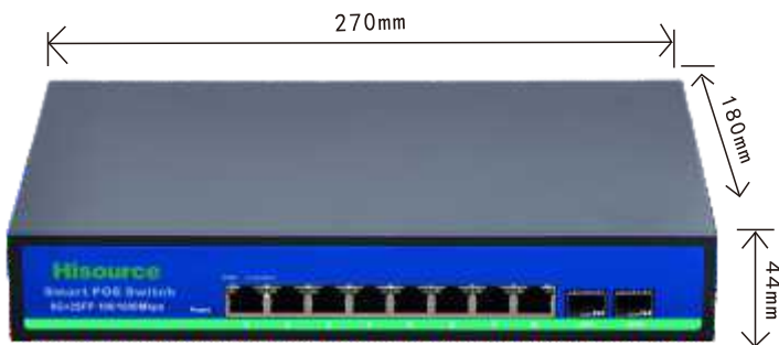
产品尺寸：270mmX180mmX44mm(L*W*H)
