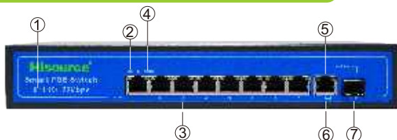
3.1: 以八口POE交换机前面板示意图3-1 (为列)
