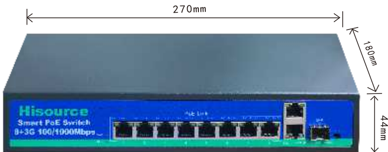
产品尺寸：270mmX180mmX44mm(L*W*H)
